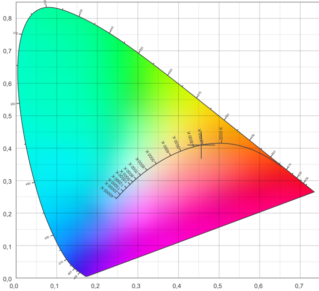
CIE 1931
